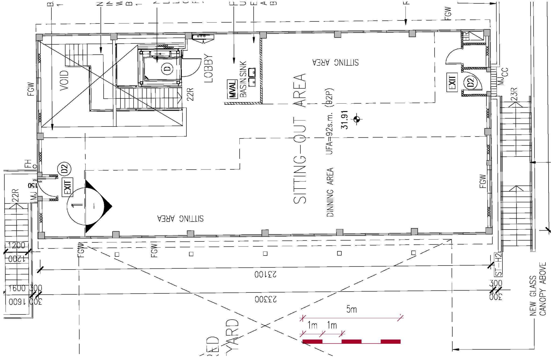
餐廳上層平面圖——餐廳上層總面積約 240 平方米，可提供約 100 個座位（該範圍約 180 平方米）。
